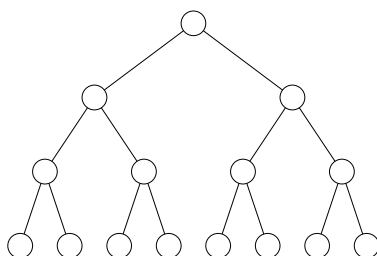
15.14. ábra. Teljes bináris fa.
